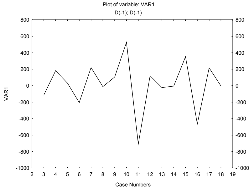
Рис. 4. Графік часового ряду других різниць
