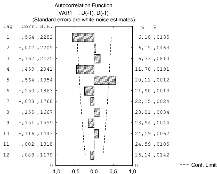
Рис. 5. Графік автокореляційної функції для ряду других різниць
